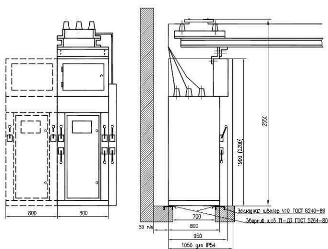
Габаритні розміри шаф КСО
